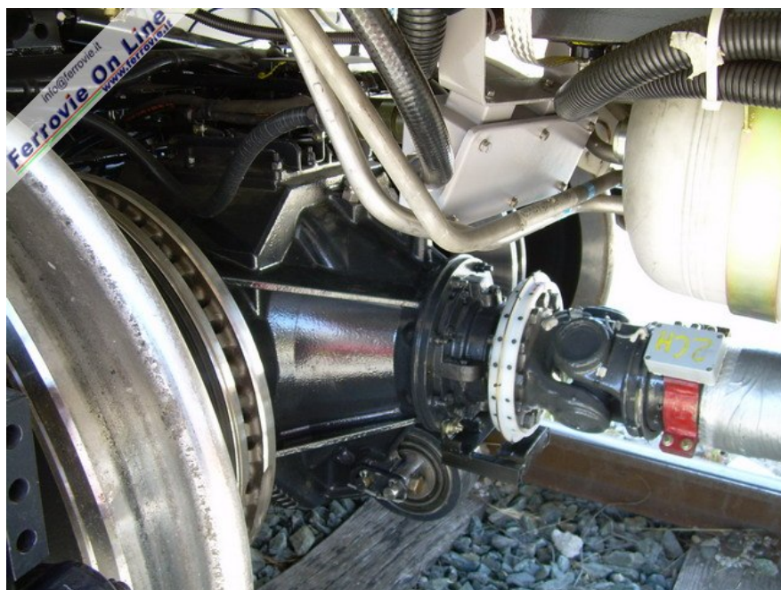
Giunto tra albero di trasmissione e carrello anteriore dell'ETR.610. (Foto Maurizio Tolini, 5 giugno 2006)
