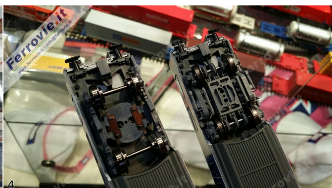
3. Carrozza doppio piano Vivalto, con carrelli Siemens SF400, di prossima consegna. 4. Dettaglio dei carrelli delle carrozze Vivalto di Vittrains: AnsaldoBreda a sinistra e Siemens a destra.
