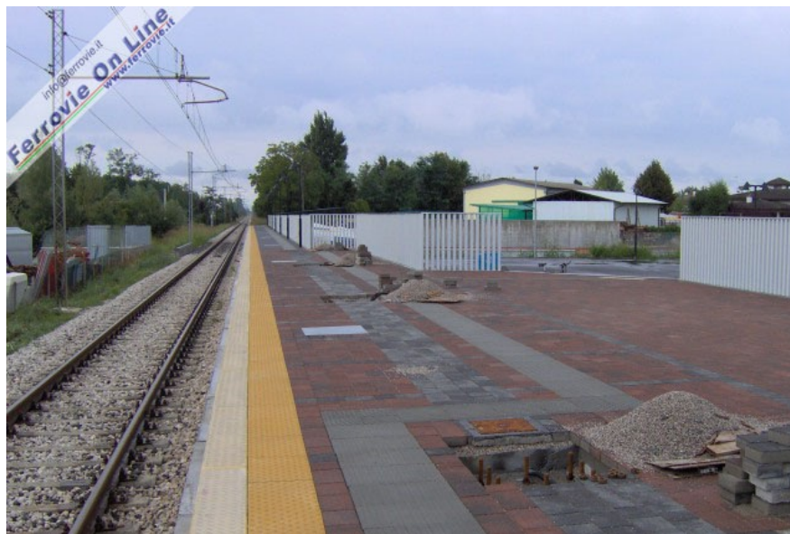
1 La nuova fermata di Trebaseleghe durante le ultime fasi dei lavori di costruzione. (Foto Riccardo Berto, 21 agosto 2005)
