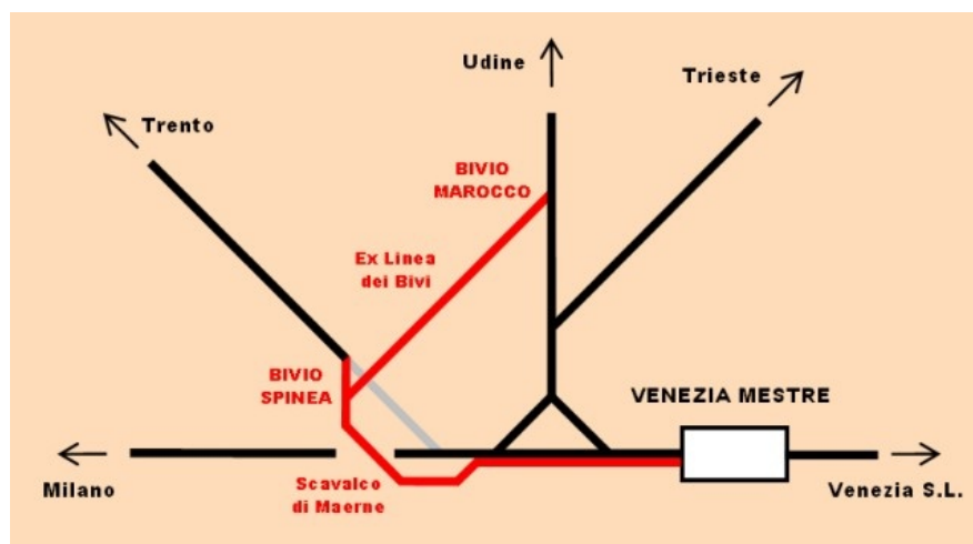
2 Schema semplificato del nodo di Mestre. In nero le linee esistenti, in rosso i tratti in fase di costruzione o ripristino, in grigio il tratto che verrà rimosso. (Disegno Fabio Veronesi)
