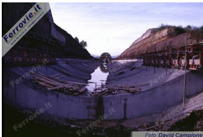
L'arco rovescio della galleria artificiale Colle Cisterna lunga 202 metri, prima della ricopertura (Foto David Campione, 31 ottobre 1997)
