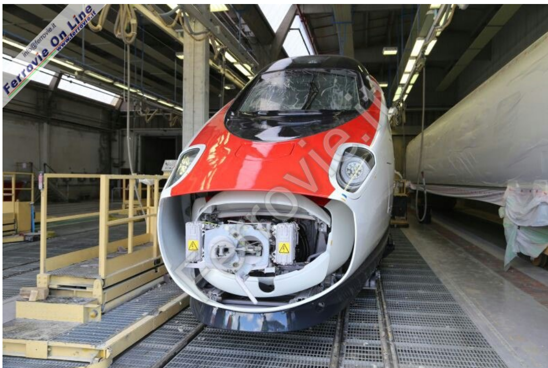
Il primo ETR.610 dell'ordine 2012 nello stabilimento Alstom di Savigliano, quasi pronto per la consegna a Ferrovie Federali Svizzere. Foto David Campione, 27 maggio 2014)
