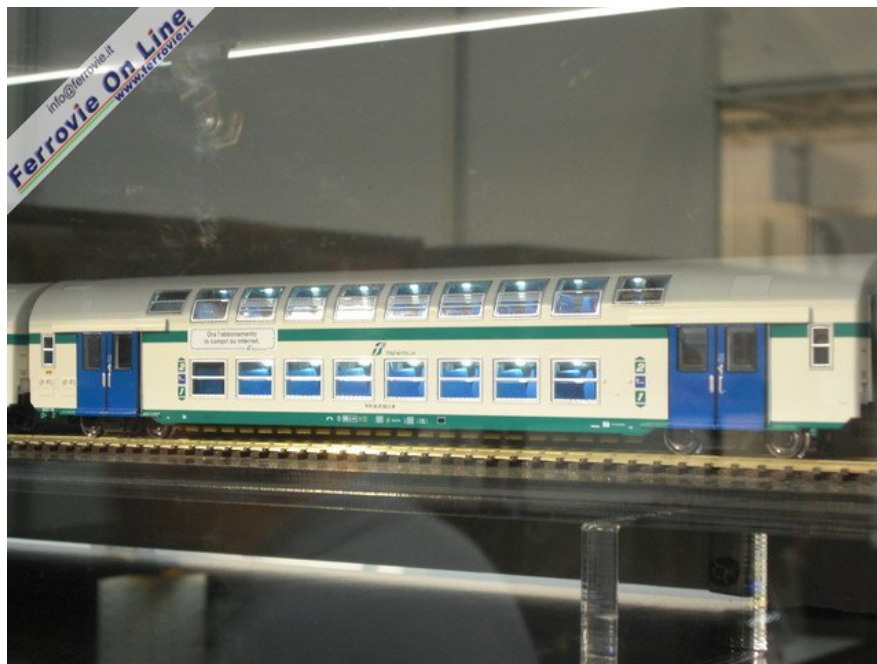
3 a Carrozza a due piani di Vitrains, già modificata con il sistema di illuminazione Almrose. (Foto David Campione)
