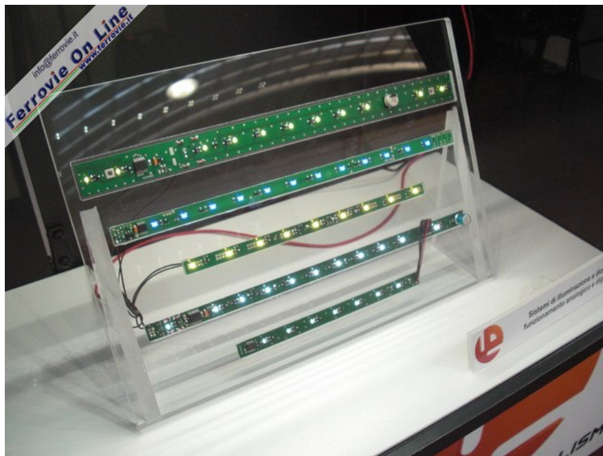
2 a Barre led di Almrose per l'illuminazione di carrozze di vario tipo. (Foto David Campione)
