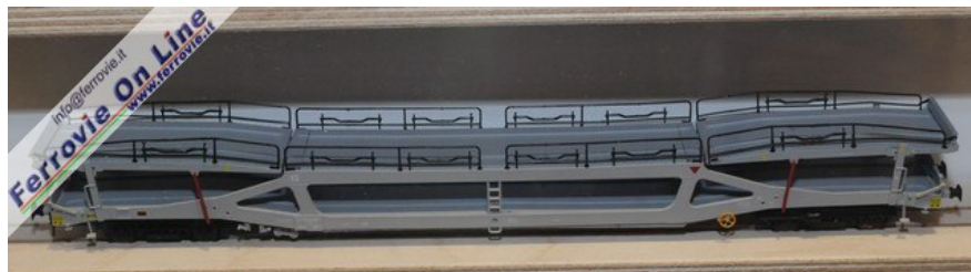
9. Campione del carro trasporto auto DDm tipo 1968 (Foto Mauro Terrone)
