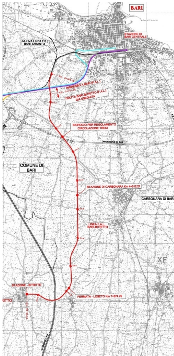
3. Tracciato della linea Bari - Bitritto
