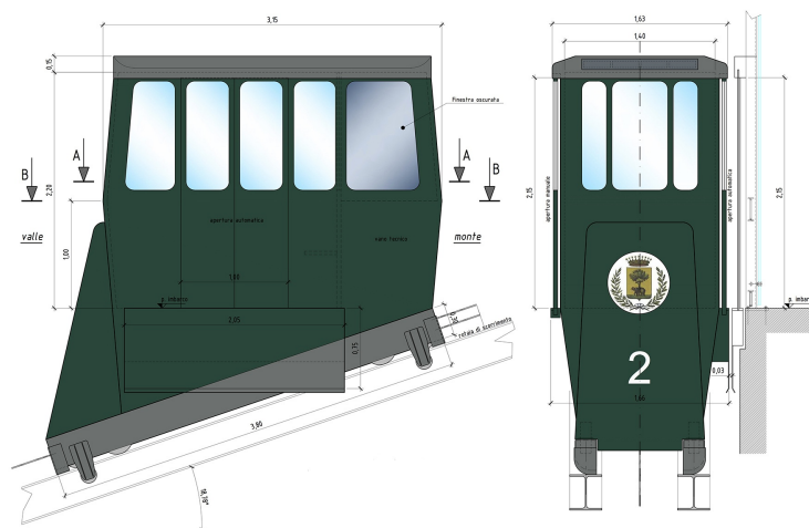
L'aspetto delle cabine della nuova funicolare del Piazzo nel progetto definitivo.
