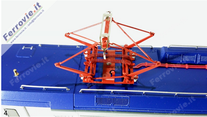
4/5. Vitraains 2208 - Locomotiva E.464.589 FS
